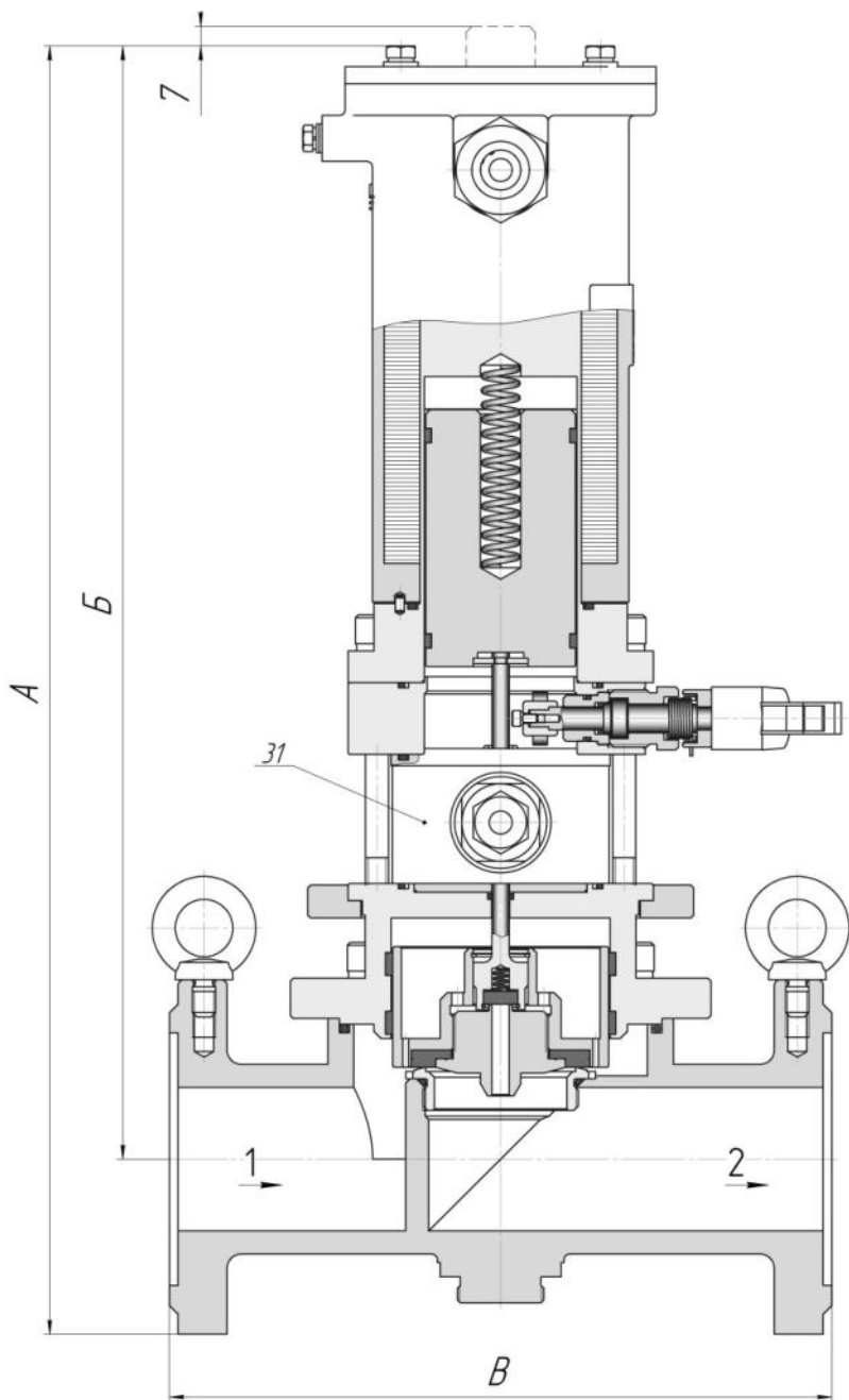
Рис. 1в. Клапан СЕНС-ПК...-ДКП. Общий вид. Остальное см. рис.1а.
