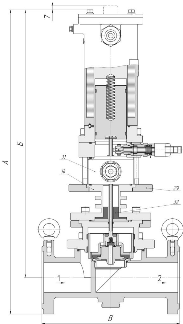
Рис. 1г. Клапан СЕНС-ПК...-200С-ДКП. Общий вид. Остальное см. рис.1а.
