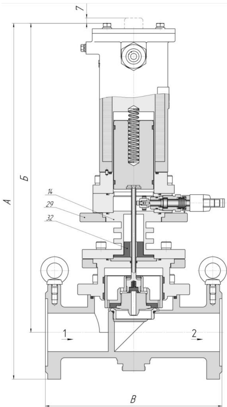
Рис. 16. Клапан СЕНС-ПК...-200С. Общий вид. Остальное см. рис.1а.
