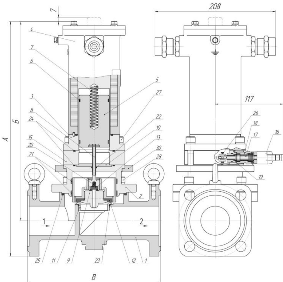
Рис. 1а. Клапан СЕНС-ПК. Общий вид.
