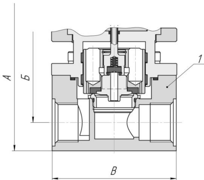
Рис. 1е. Вариант исполнения клапана DN25 с муфтовым присоединением. Остальное по рисунку 1а, б, в, г
