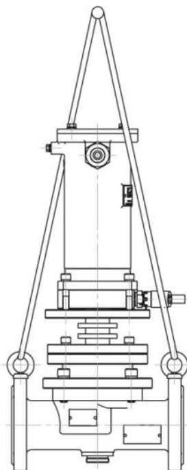
Рисунок 7 – Схема строповки клапана
