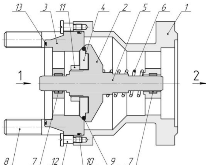
Рис. 2. Устройство обратной герметичности УОГ
